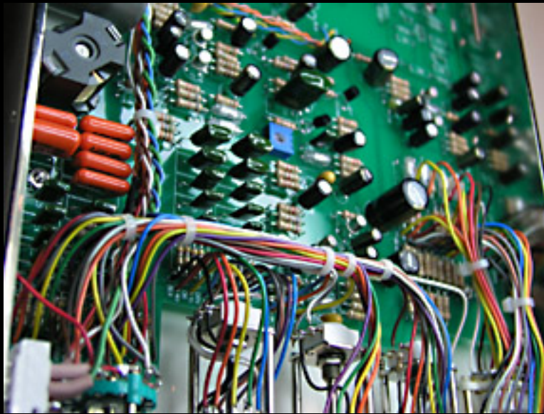
inside module
